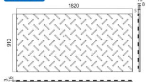
FW36 (厚型)
