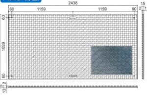
FW48 (厚型)
