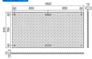
FW36 (厚型)
