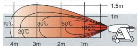
●温度分布図(上昇温度0°C基準)
